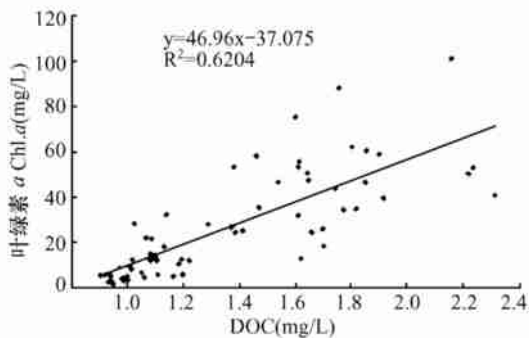
图4 香溪河库湾 Chl. a 与 DOC 浓度回归分析
