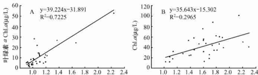
图5 不分阶段 Chl. a 与 DOC 浓度回归分析
